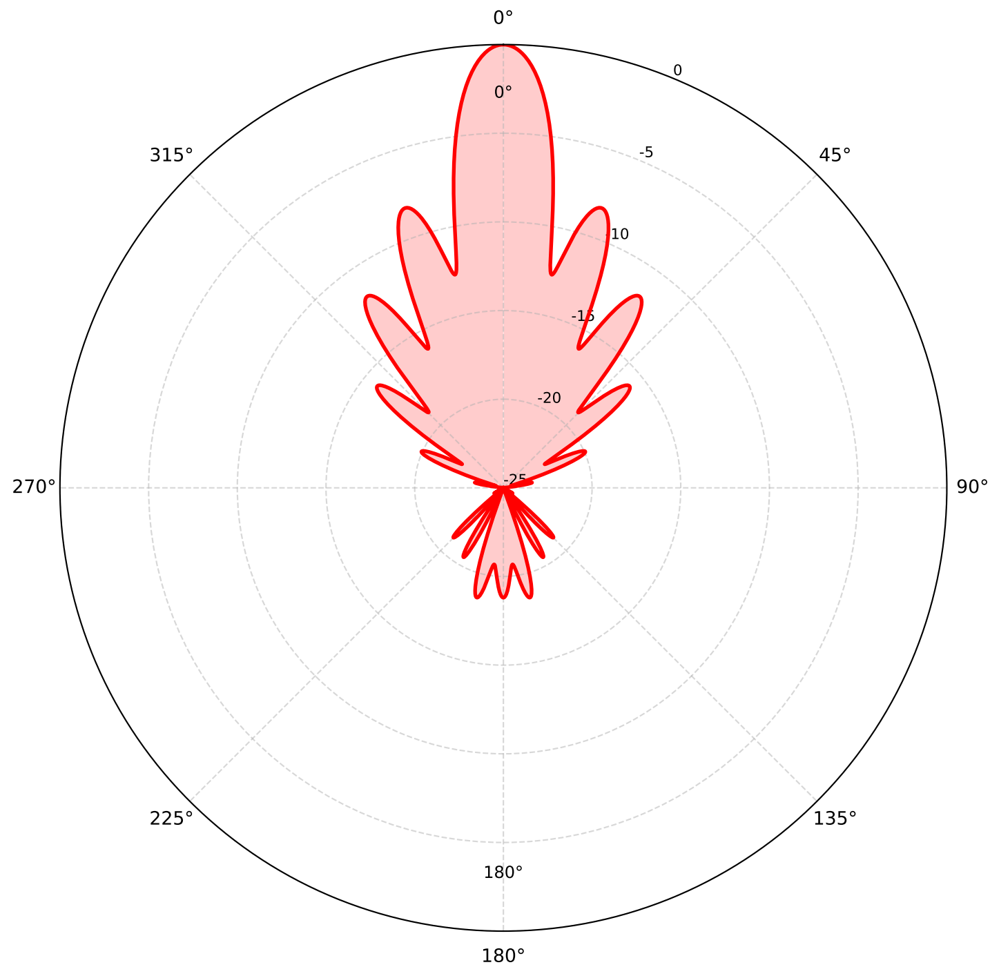
Рассеяние Ми, лог. шкала
